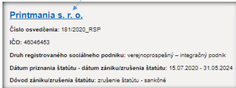
Obrázok 27 - základné informácie
