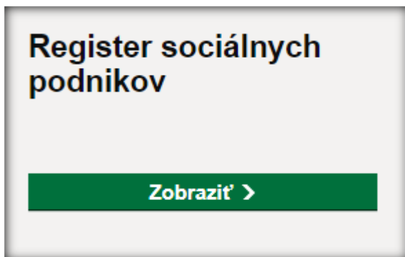
Obrázok 2- tlačidlo Zobraziť
